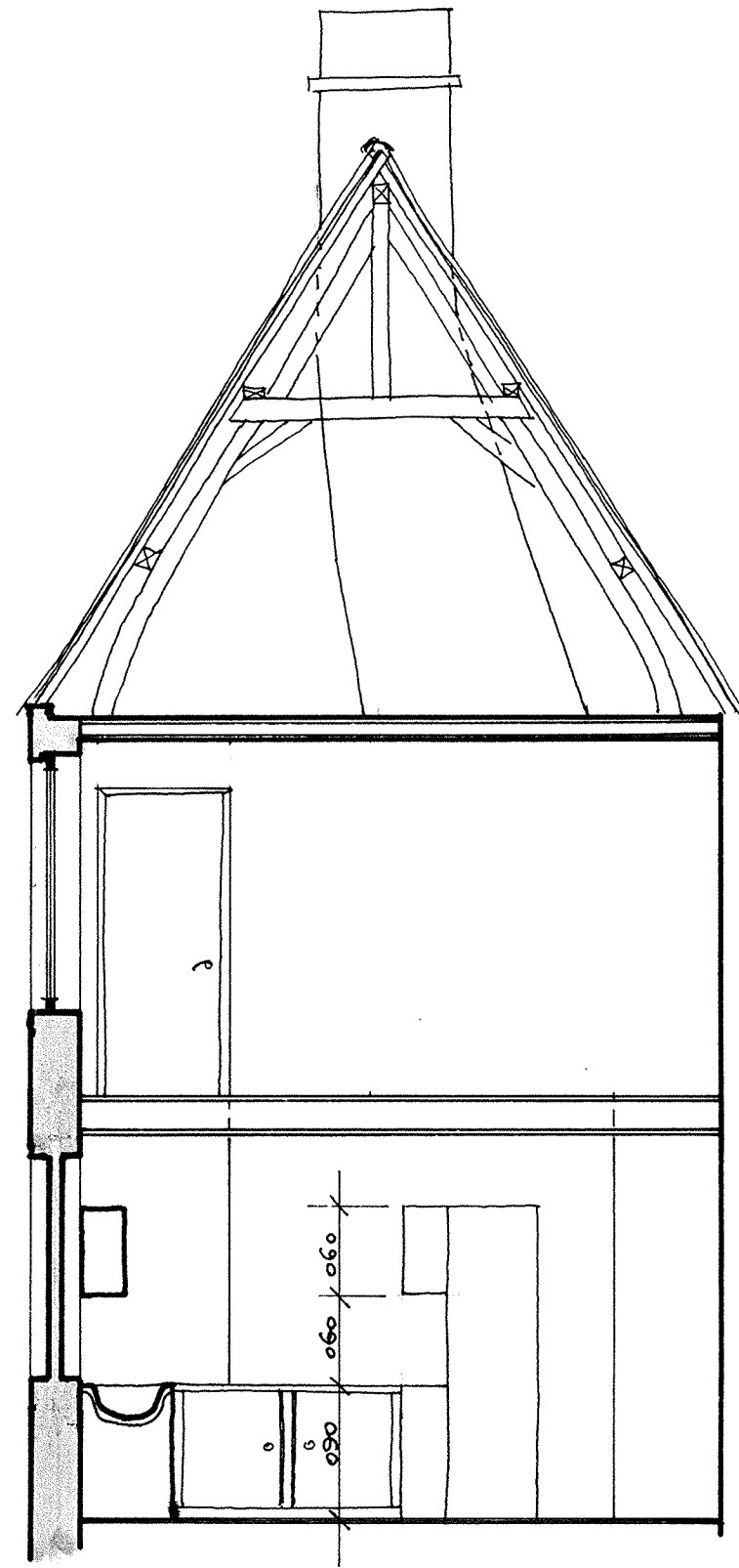
DOORSNEDEN A-A
