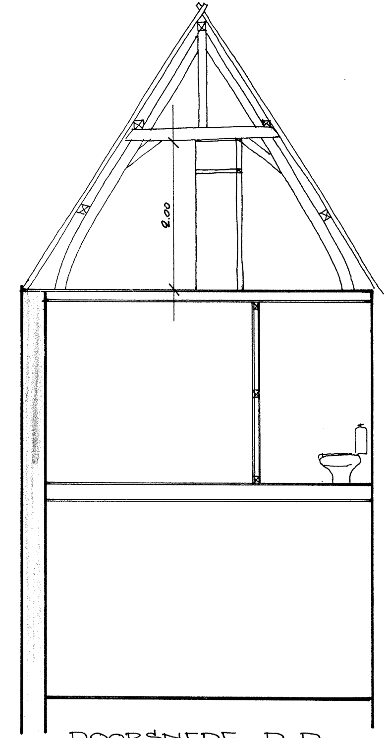
DOORSNEDEN D-D
