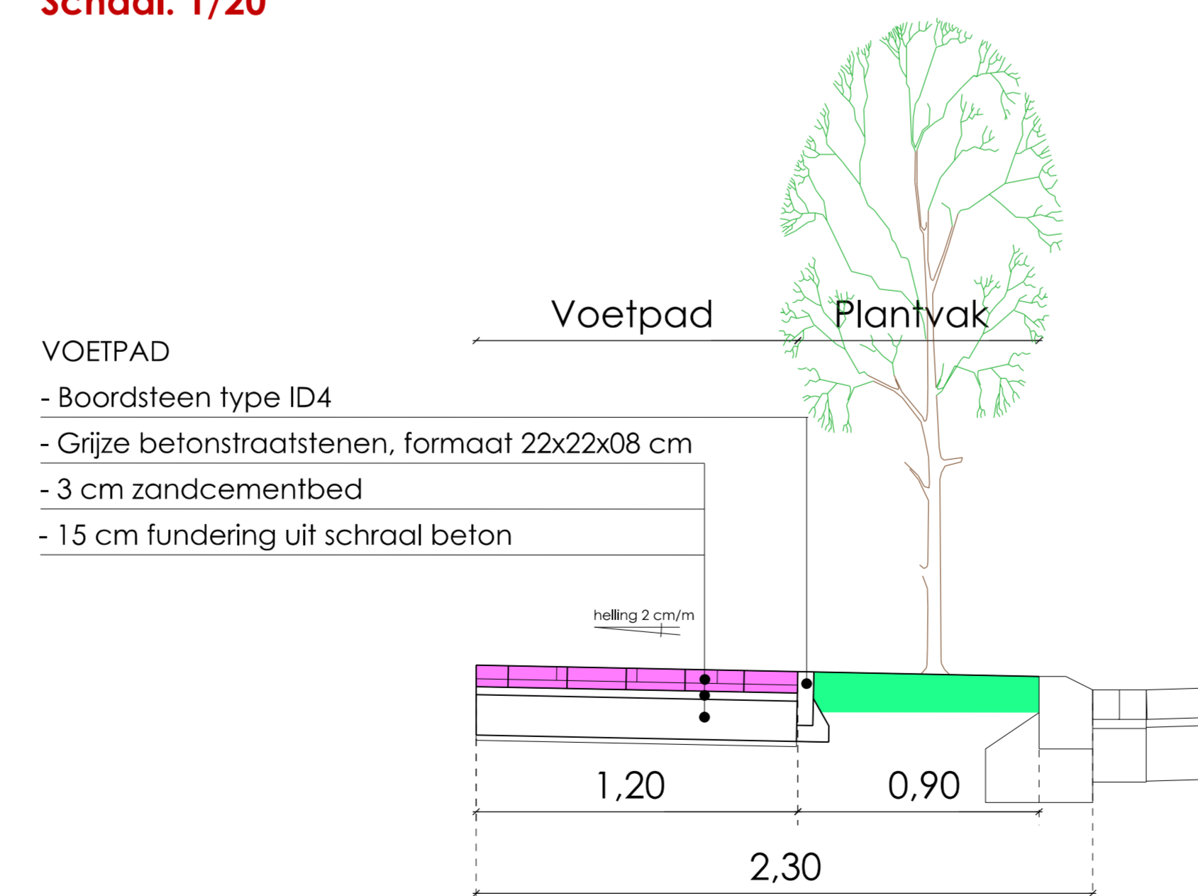
Dwarsprofiel ontwerp B-B' Schaal: 1/20
