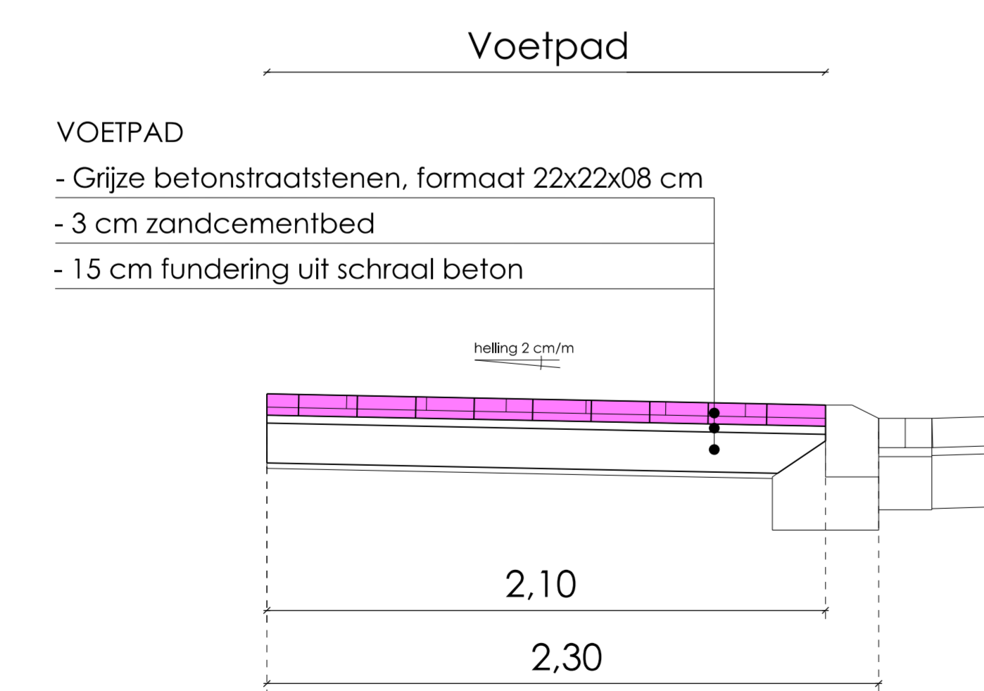
Dwarsprofiel ontwerp A-A' Schaal: 1/20
