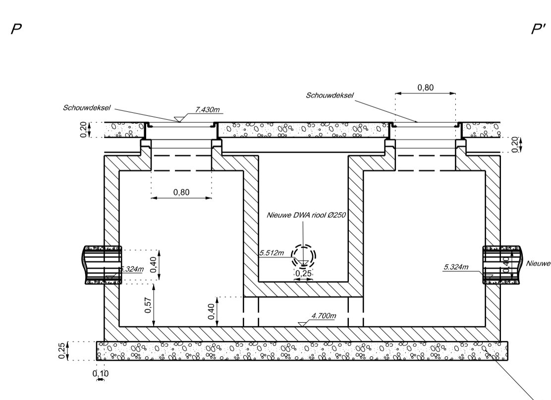
Detail 1: ter plaatse gemaakte of geprefabriceerde sifonput RWA93
